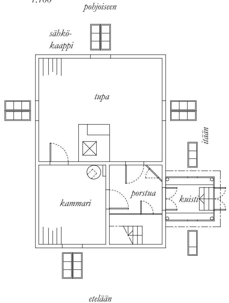
Pohjapiirros, asuin kerros 1:100
