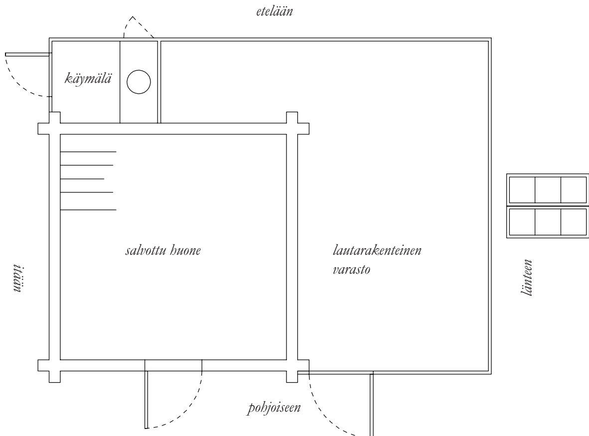
Pohjapiirros, liiteri 1:50
